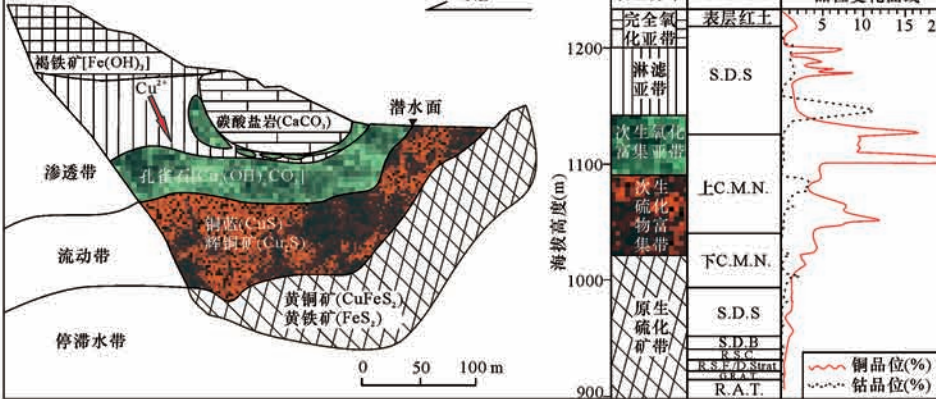
(b) 表生成矿富集机制
